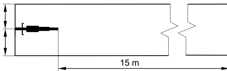
3. ábra: A jármű bolyozási zóna (egyenlő nyomon haladó járműveknél)
