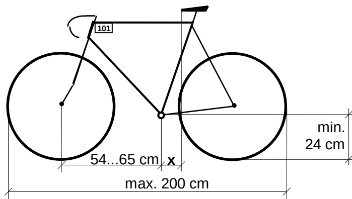
1. ábra: A kerékpár méretei
