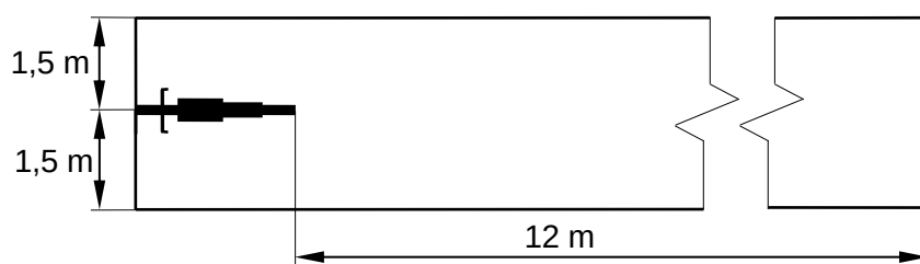
3. ábra: A jármű bolyozási zóna (egy nyomon haladó járműveknél)
