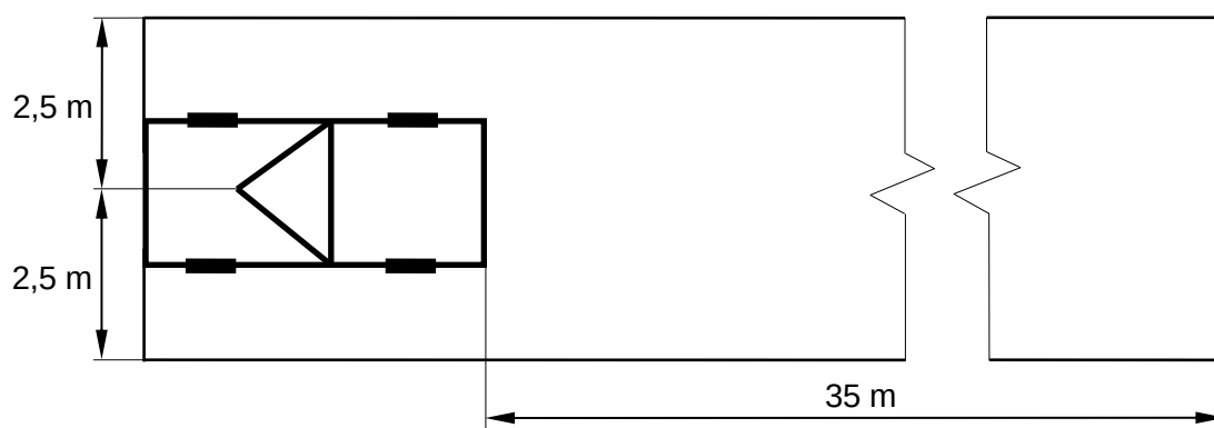
4. ábra: A jármű bolyozási zóna (több nyomon haladó járműveknél)
